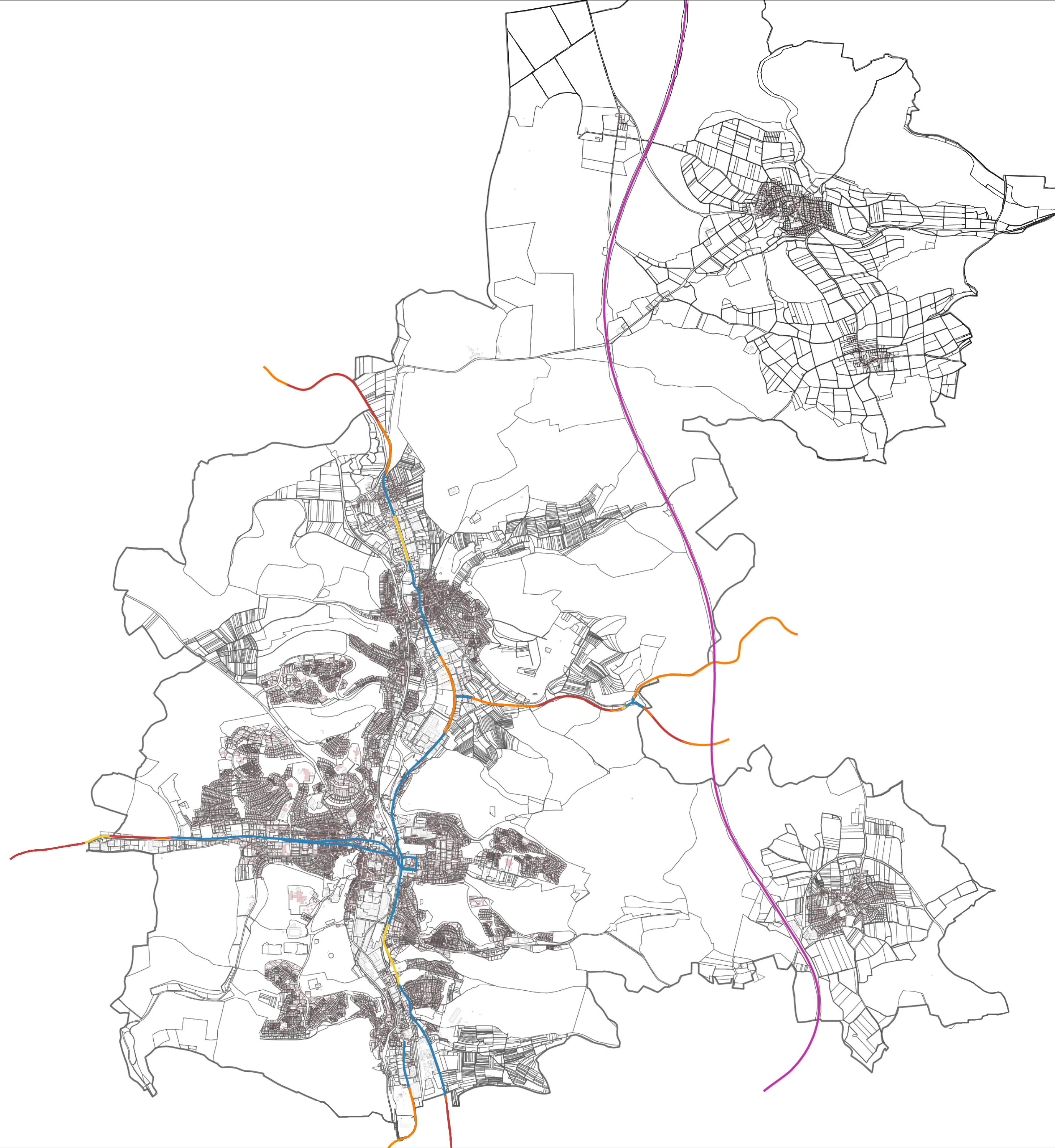
Geschwindigkeitenkarte Ist-Zustand
